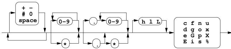
Рис. 1: Синтаксис спецификаций преобразования функции printf (C90)
